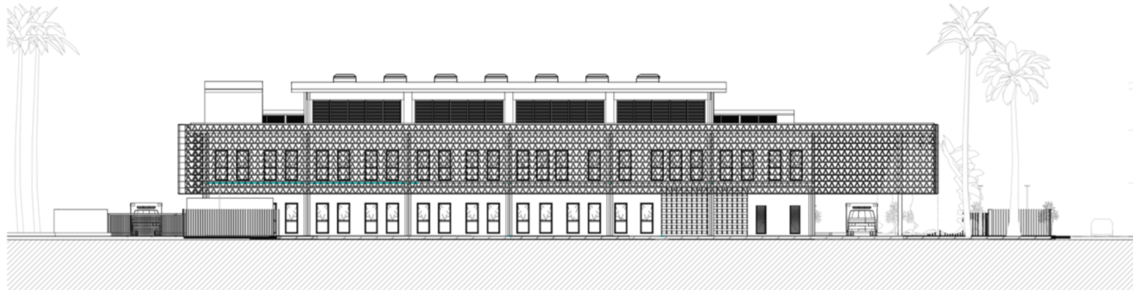
Facade Nord Ech : 1 : 300
